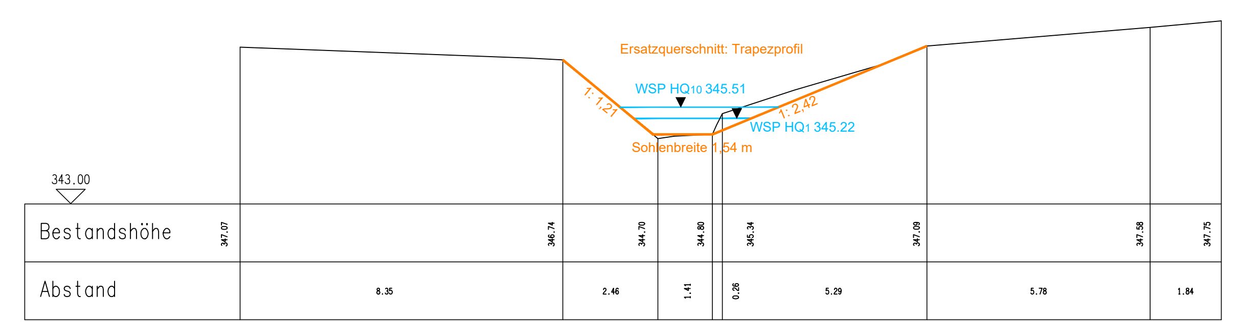
Schnitt B - B
